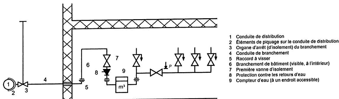
Figure 2 : Schéma type d'un branchement d'immeuble
