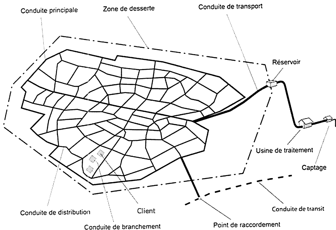
Figure 1 : Schéma de principe du réseau d'eau potable.
