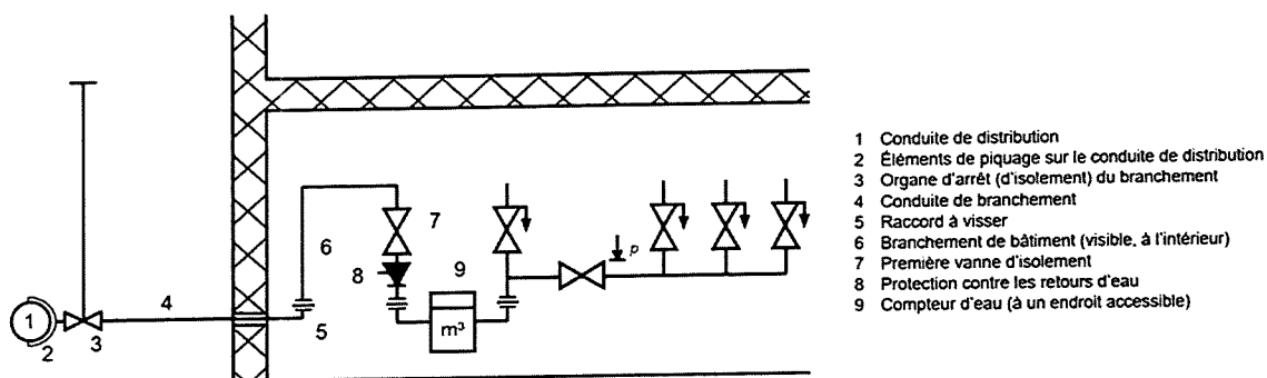
Figure 2 : Schéma type d'un branchement d'immeuble
